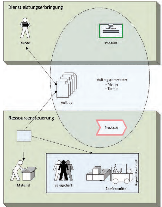
Modell Auftragsmanagement
